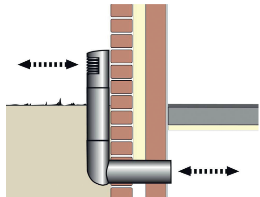
Extra grote luchtdoorlaat met het grootste model Ross ventilatieschacht van \varnothing 200\text{mm} !
