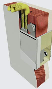
IN DE WAND GEÏNTEGREERDE INBOUW U 2 MET KANAALAANSLUITING
