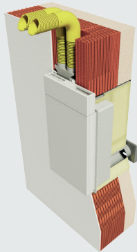
INBOUWUITVOERING MET KANAALAANSLUITING
